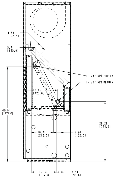
50BRN,BZN016
