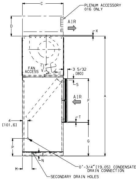
LEFT SIDE
