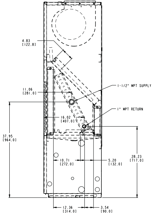
50BRN,BZN006,008
