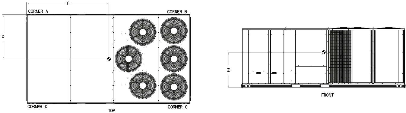
Fig. 10 - 50TC*D30
