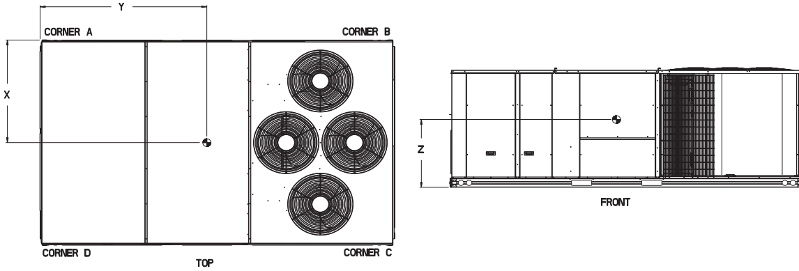
Fig. 6 - Dimensions 50TC-D24-28
