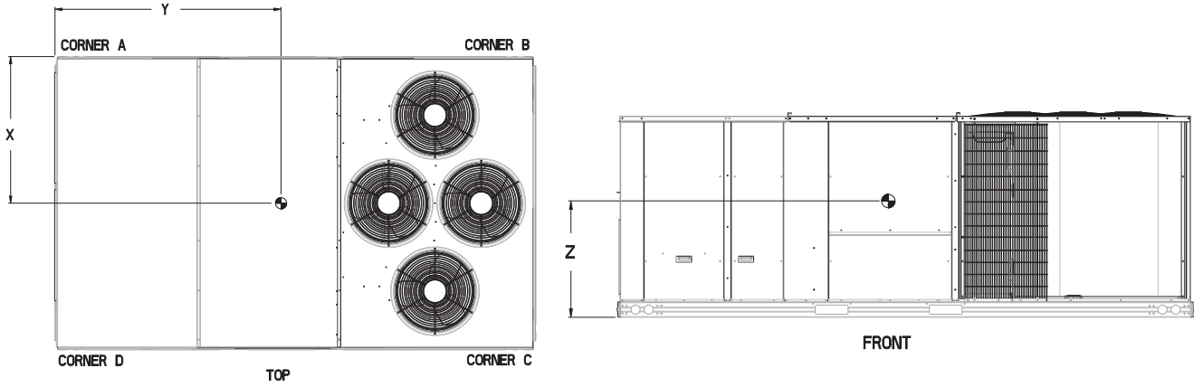
Fig. 6 - Dimensions 50TCQD24-28
