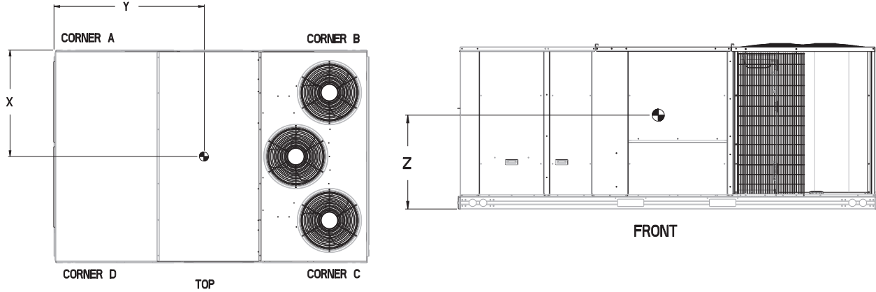
Fig. 2 - Dimensions 50TCQ-17
