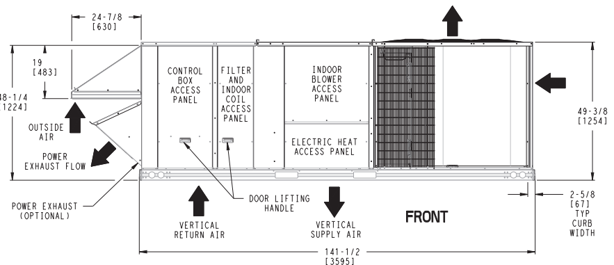
Fig. 5 - Dimensions 50TCQ-24
