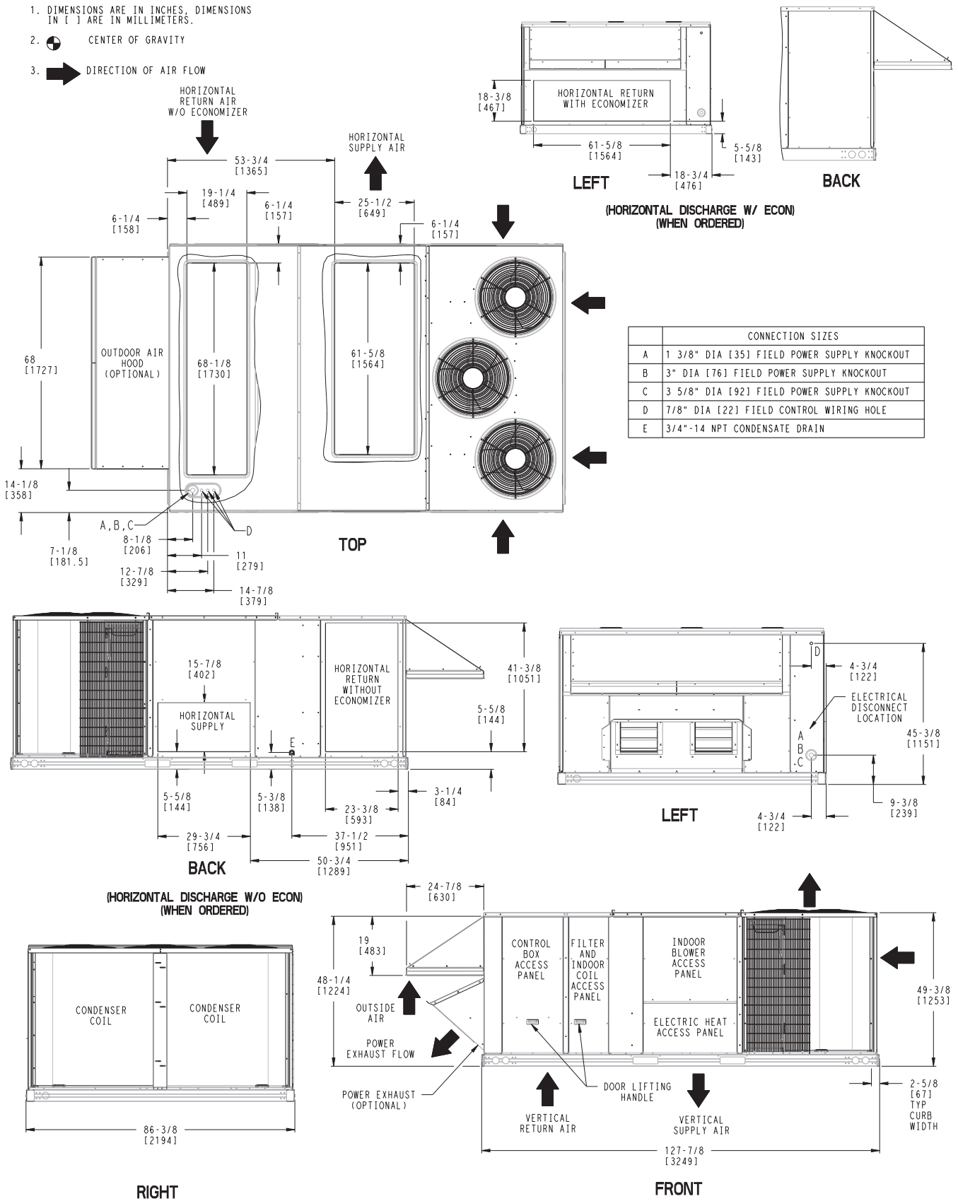
Fig. 1 - Dimensions 50TCQ-17
